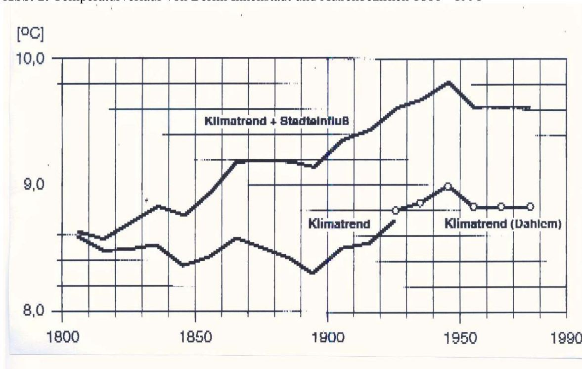
Abb. 1: Temperaturverlauf von Berlin Innenstadt und Außenbezirken 1800 - 1990
