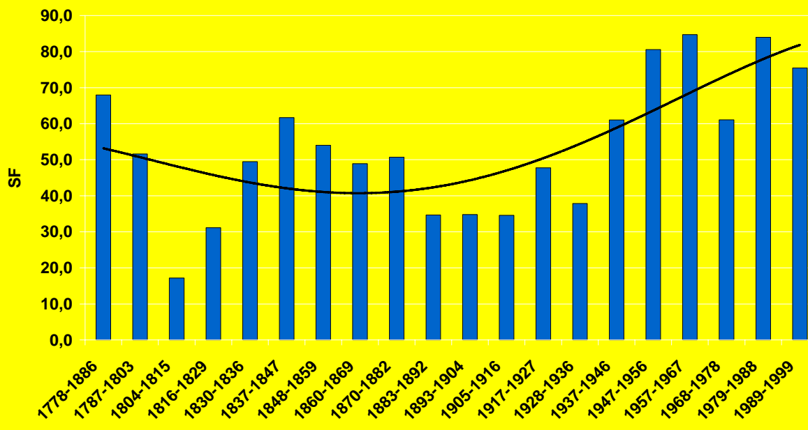
Abb.5 Mittlere Sonnenfleckenanzahl je Zyklus 1778 - 1999
