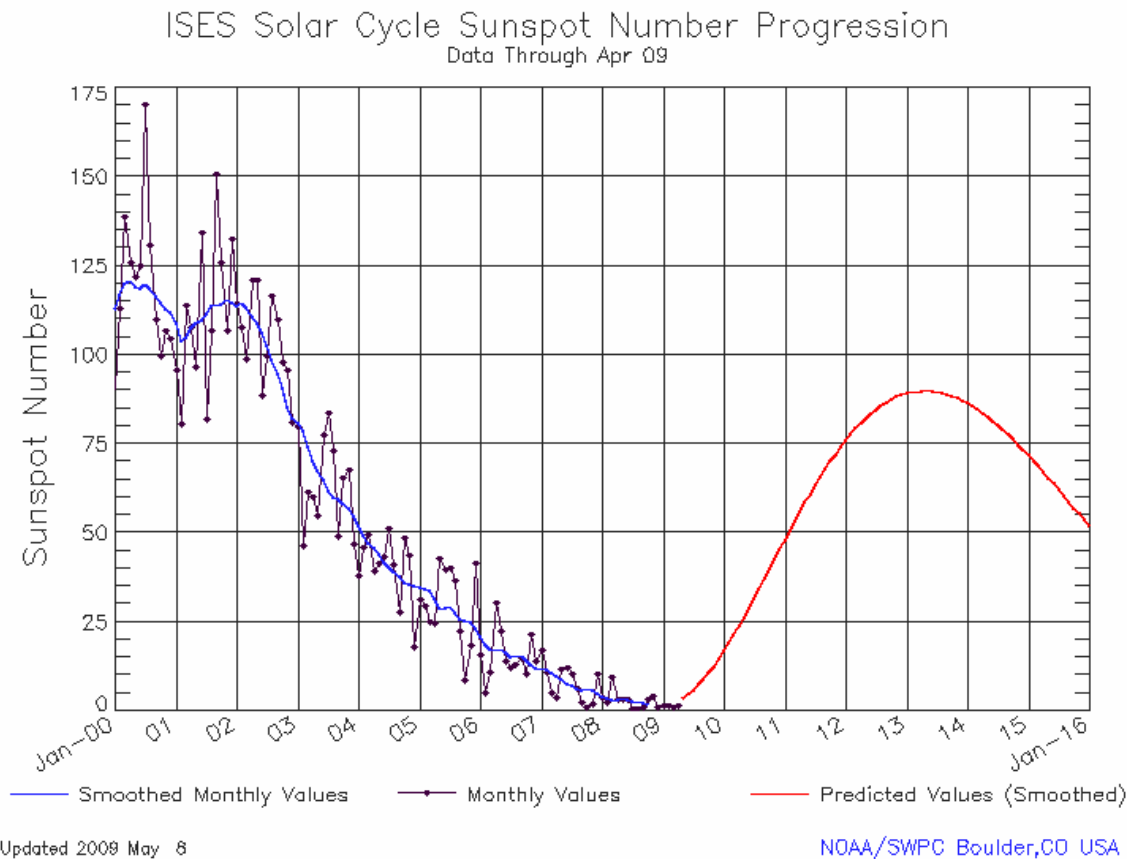
Abb.8: Verlauf des 23. und Vorhersage des 24. Sonnenfleckenzyklus (NOAA)
