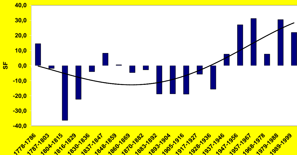
Abb.7 Abweichung der mittleren Sonnenfleckenanzahl je SF-Zyklus vom Durchschnitt 1778 - 1999
