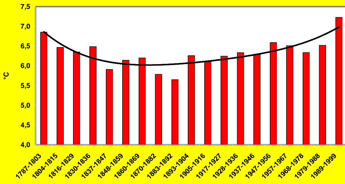
Abb.4 Mitteltemperatur je Sonnenfleckenzyklus von Hohenpeißenberg 1787 - 1999
