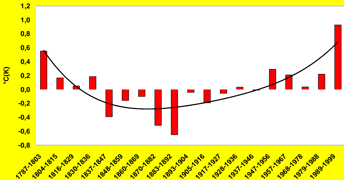
Abb.6 Mittlere Temperaturabweichung je Sonnenfleckenzyklus vom Durchschnitt 1787 - 1999
