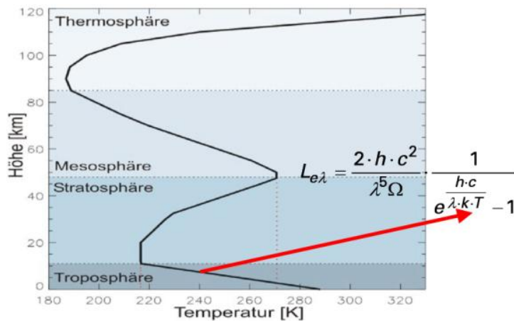
Bild 7: Strahlungstransport, Planck-Gleichung und gemessener Temperaturgradient
