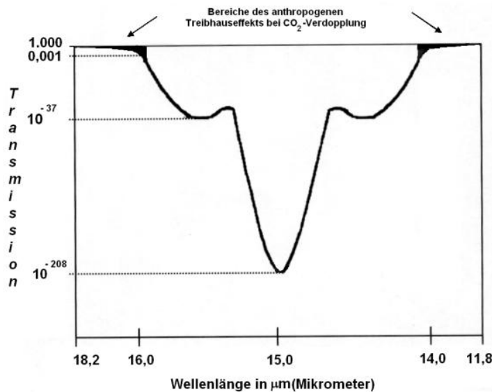
Bild 3: Spektrales Auswertungsschema
