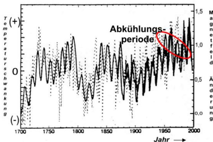
Bild 11: Solares Magnetfeld und Globaltemperatur (abgewandelt nach 28)
