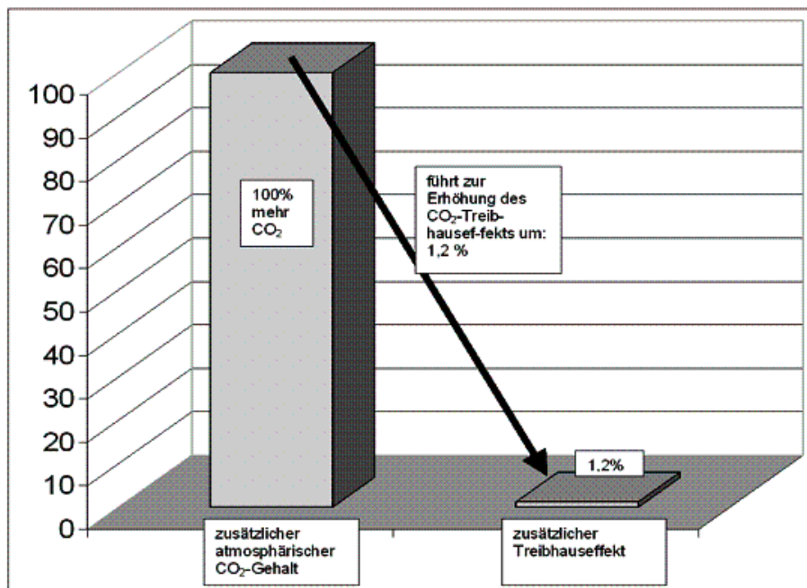
Bild 4: Prozentuale Erhöhung des Treibhauseffekts bei Verdopplung des atmosphärischen CO 2 -Gehalts gemäß der offiziellen Angaben des IPCC
