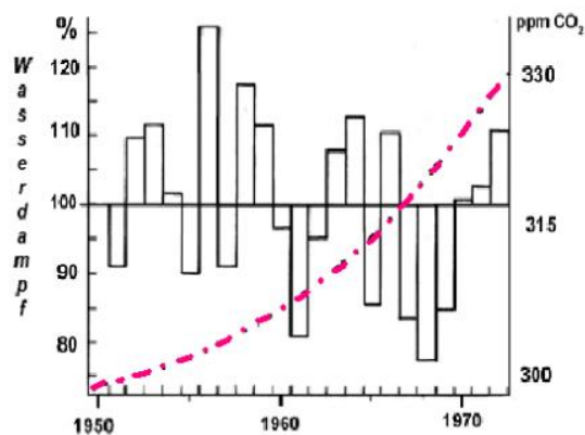
Bild 5: Prozentuale Abweichung des Wasserdampfgehalts über dem Atlantik (33)
