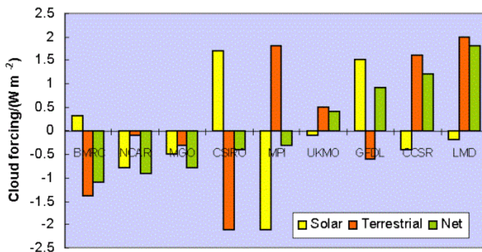
Bild 9: Strahlungsantrieb der Wolken mit unterschiedlichen Klimamodellen gerechnet
