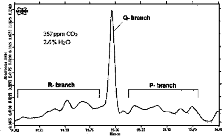
Bild 2: Unbearbeitetes Spektrum der 15 \mu\text{m} -Bande ( n_2 -Bande)
