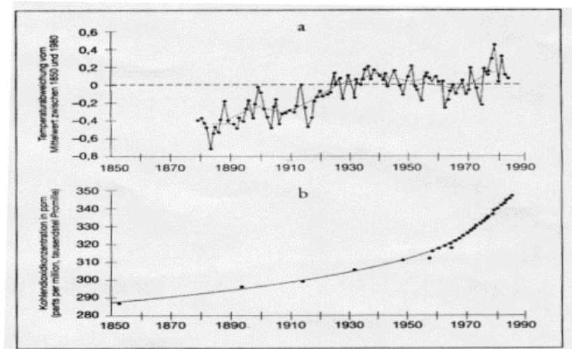
Bild 10: CO 2 -Gehalt und Temperaturverlauf (vgl. a. Bild 11)
