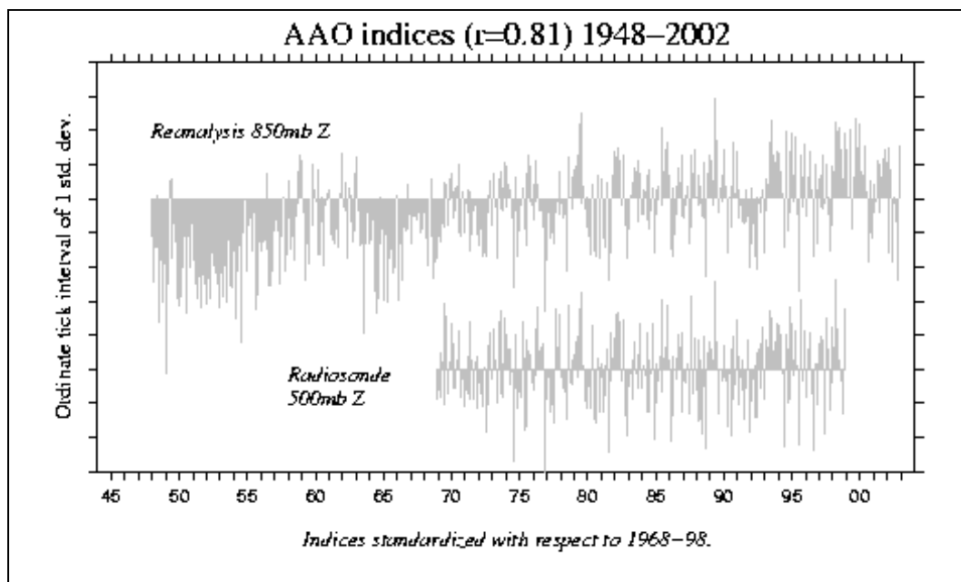
Abb.3 [10] Antarktische Oszillation (AAO)
