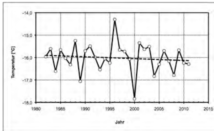
Abb.5 [14] Temperatur-Abkühlungs-Trend an der NEUMAYER-Station
