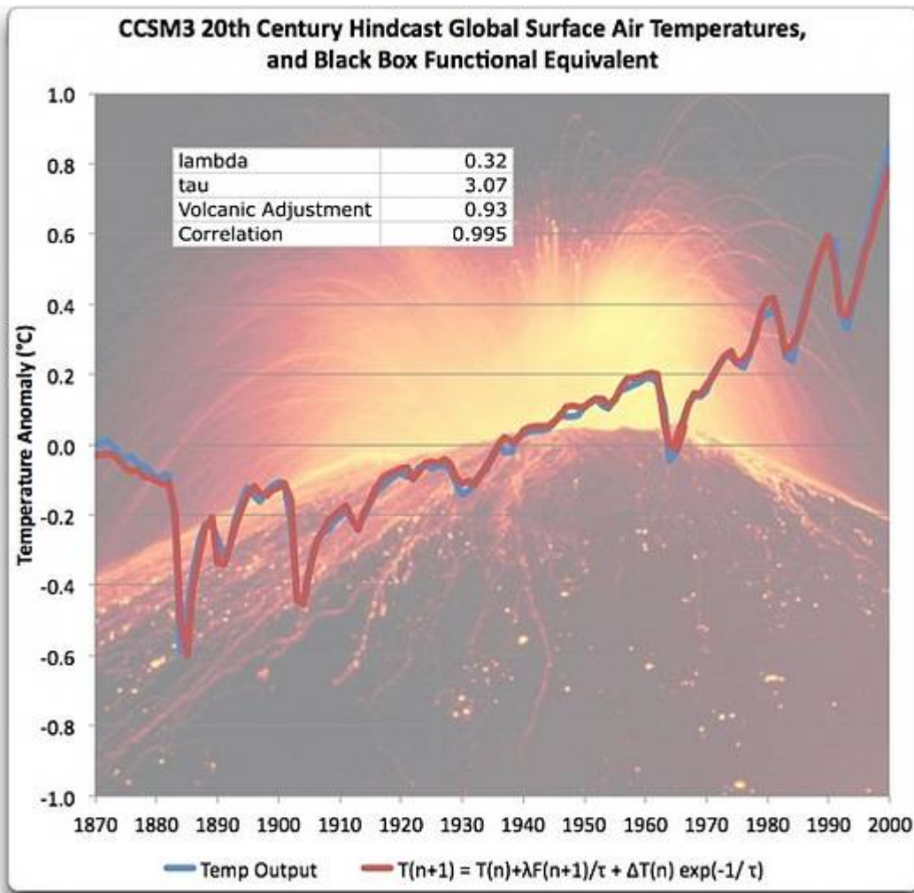
Abbildung 3. Gleichung zum funktionalen Äquivalent des CCSM3-Klimamodells im Vergleich zum aktuellen Output von CCSM3. Beide sind etwa identisch.
