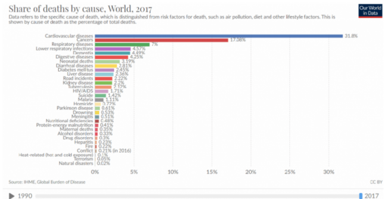
Bild 6 Anteilige Mortalität von Umwelteinflüssen weltweit (Heat-related: 0,1 %)
