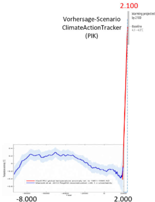
Bild 17 Verlauf Marcott et al (2013) und ClimateActionTracker Projektion Baseline. Vom Autor zusammengestellt
