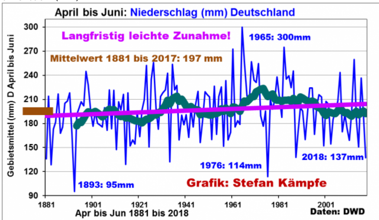
Abbildung 5: Langfristig wurde es von April bis Juni in Deutschland eher feuchter. Das Gebietsmittel 2018 liegt mit 137 mm zwar deutlich unter dem Langjährigen Mittel von 197mm (brauner Balken); schaffte es aber nicht unter die trockensten fünf dieser Zeiträume seit 1881.
