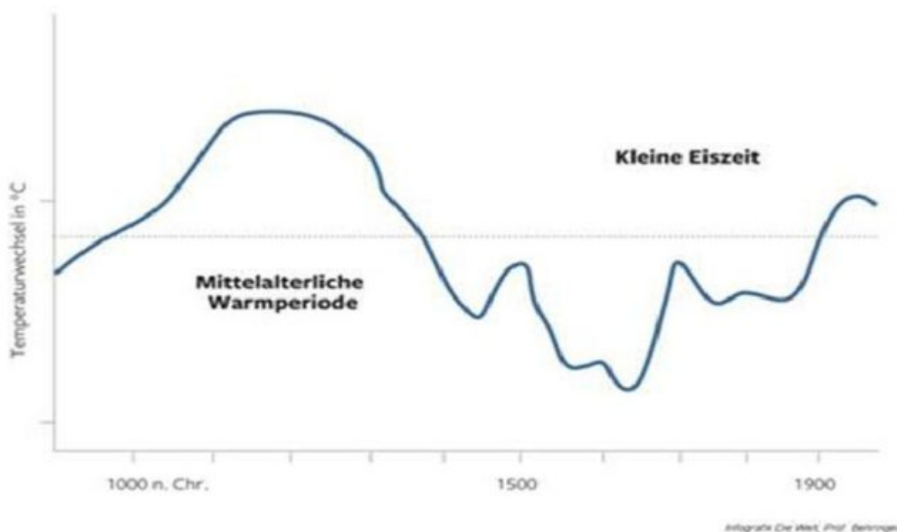
Abb. 6: Der Temperaturverlauf Europas in den letzten 1100 Jahren. Von einer mittelalterlichen Warmzeit, als die Alpen weitgehend gletscherfrei waren, sind wir noch lange entfernt. Am rechten Ende sieht man ab 1850 die Beendigung der kleinen Eiszeit, 1900 erreichen wir wieder die 1100-jährige Durchschnittsline. Seit 1998 ist der fallende Trend erkennbar. Die letzten 120 Jahre müssten allerdings noch WI-bereinigt werden, siehe unsere Abb. 4.
