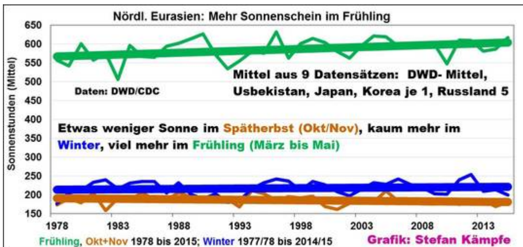
Abbildung 6: Die nicht repräsentative Mittelung aus 9 Stationen weist auf eine geringe Abnahme der Sonnenscheindauer im Spätherbst um etwa 10 Stunden, aber auf eine merkliche Zunahme im Frühling um etwa 37 Stunden, hin. Alle 3 Frühlingsmonate wurden sonniger, besonders der März und der Mai.
