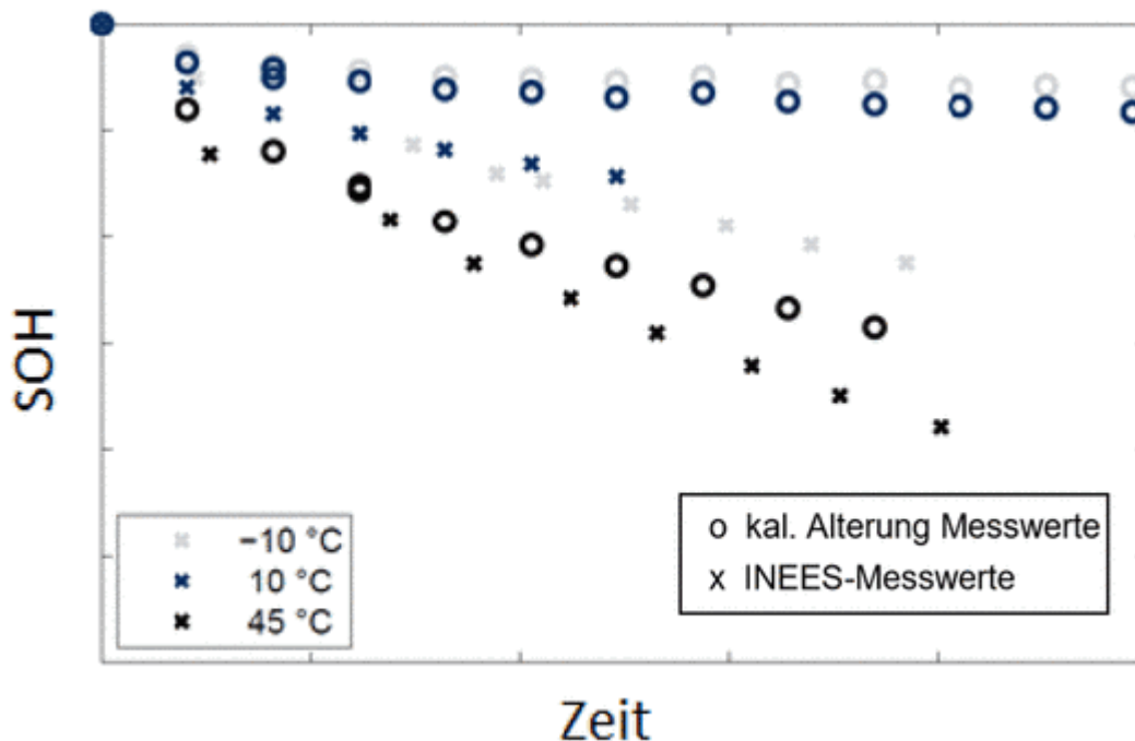
Abbildung 59: Vergleich der Alterung durch reine Lagerung und durch SRL-Profil
