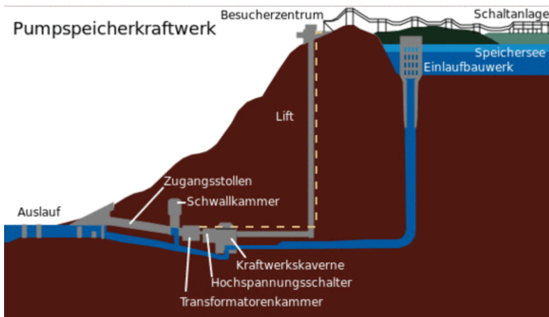
Bild 2. Schemadarstellung eines Pumpspeicherkraftwerks (Racoon Mountain) (Grafik: Wikipedia)
