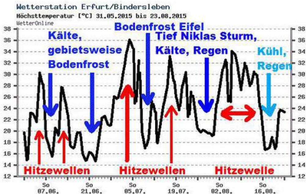
Abb. 3: Verlauf der Maximum- Werte in Erfurt vom 31.05. bis zum 23.08.2015 (Quelle: wetteronline.de, nachbearbeitet von Stefan Kämpfe). Im Juni/Juli wechselten sehr kühle mit sehr warmen Abschnitten, wobei im Juni die Kälte überwog. Nur in der ersten Augushälfte gab es mit kleinen Abstrichen über längere Zeit beständiges, sehr warmes Wetter. In der ersten Sommerhälfte wurden ungewöhnlich häufig Bodenfröste gemeldet, im Juni mehrfach in Norddeutschland, am 10. Juli in der Eifel.
