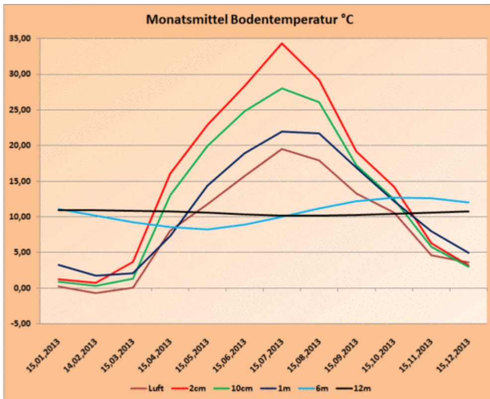
Bild 3. Jahrgang der Temperatur in der Luft sowie im Erdboden im Jahre 2013. Bei 12 m ist faktisch nur noch der Gesamt-Jahreseinfluss zu erkennen (Daten: WIKI und PIK, Grafik: Autor)
