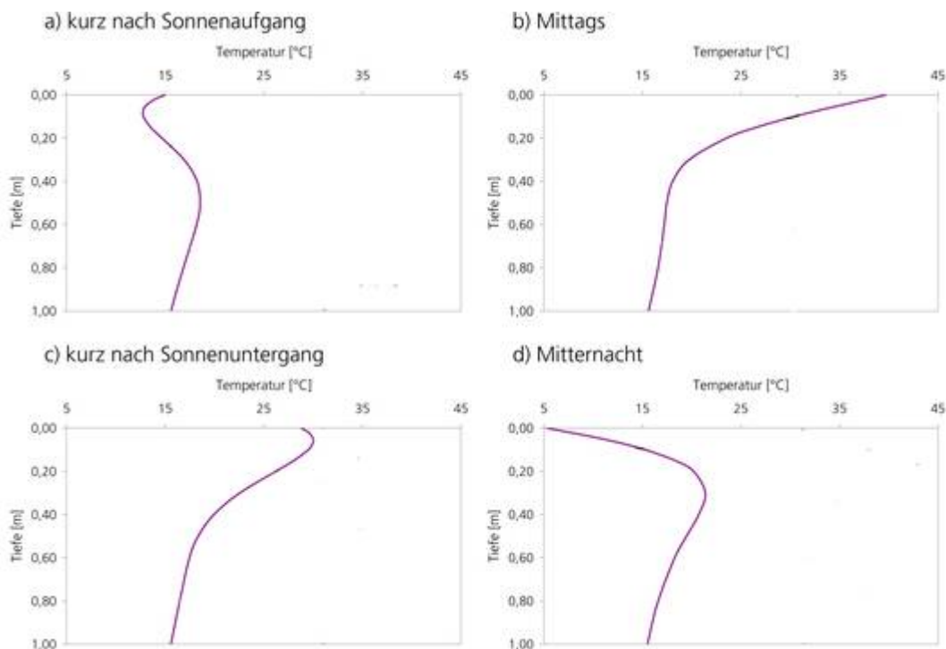
Bild 2. Tagesgang der Temperaturprofile im Boden zwischen Oberfläche und 1 m Tiefe an einem typischen Sommertag [BAYE]
