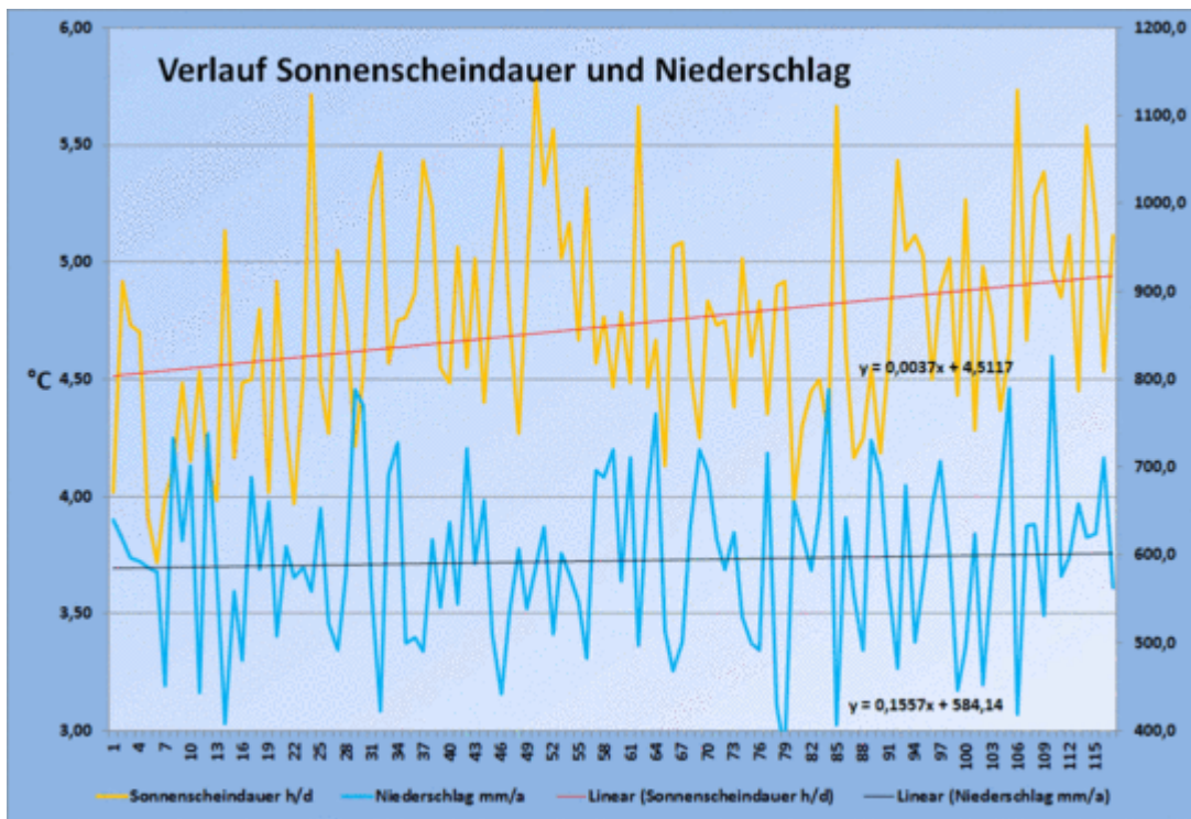
Bild 5. Während die mittlere Sonnenscheindauer in Deutschland den letzten 116 Jahren deutlich zugenommen hat, sind die Niederschlagsmengen nahezu unverändert geblieben (Daten: PIK, Grafik: Autor)
