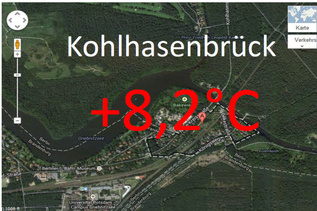
Abb.9d zeigt die Satellitenaufnahme von der Umgebung, in der die Messstation Kehlhasenbrück lag und den durchschnittlichen Jahreswert der Temperatur im Betrachtungszeitraum 1970-1974.
