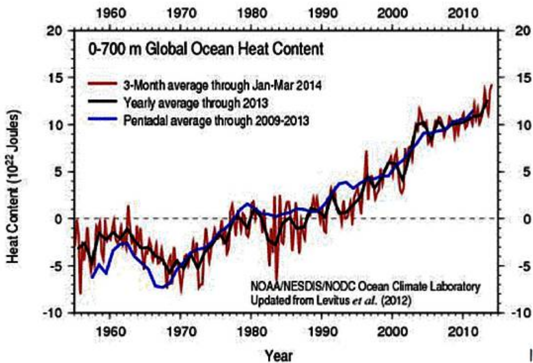
Abbildung 2: Entwicklung des ozeanischen Wärmehalts für die letzten 60 Jahre (Tiefenintervall 0-700m). Quelle: NOAA .
