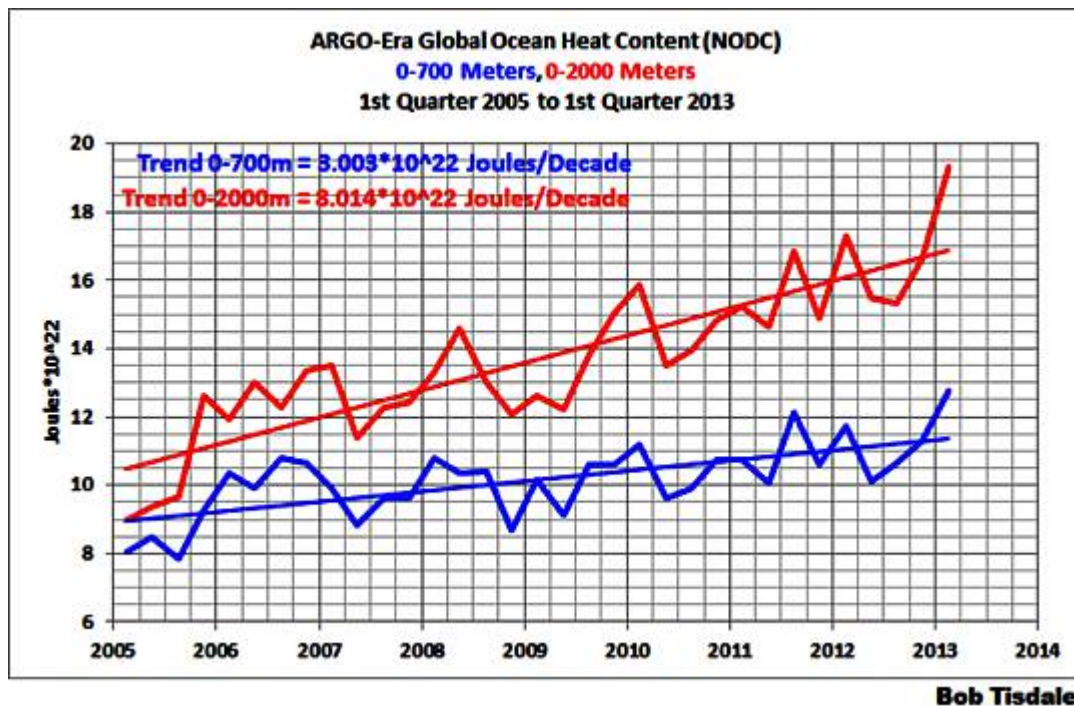
Abbildung 6: Entwicklung des OHC für die beiden Tiefenbereiche 0-700m und 0-2000m in den letzten 10 Jahren. Daten: NODC, Graphik: Bob Tisdale .
