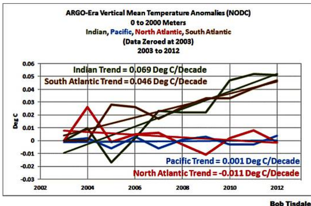
Abbildung 11: OHC-Trends aus der Argo-Ära, aufgeschlüsselt auf die wichtigsten Ozeane. Daten: NODC, Graphik: Bob Tisdale
