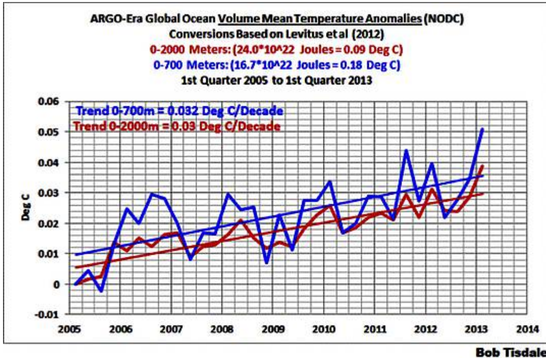
Abbildung 7: Globale Temperaturentwicklung der Meere für die beiden Tiefenbereiche 0-700m und 0-2000m in den letzten 10 Jahren. Daten: NODC, Graphik: Bob Tisdale .
