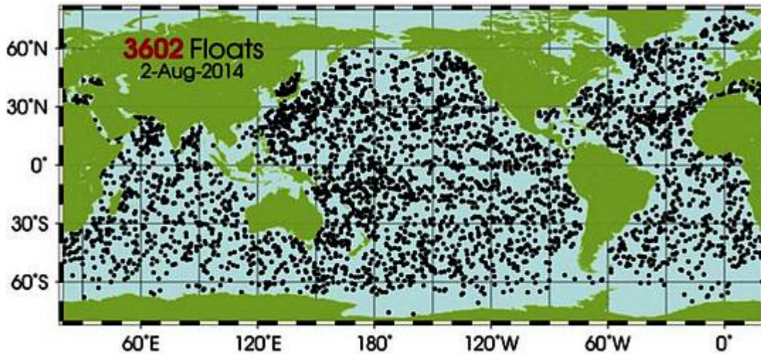
Abbildung 1: Lagekarte der Argo-Bojen am 2. August 2014. Abbildung: Argo-Webseite .
