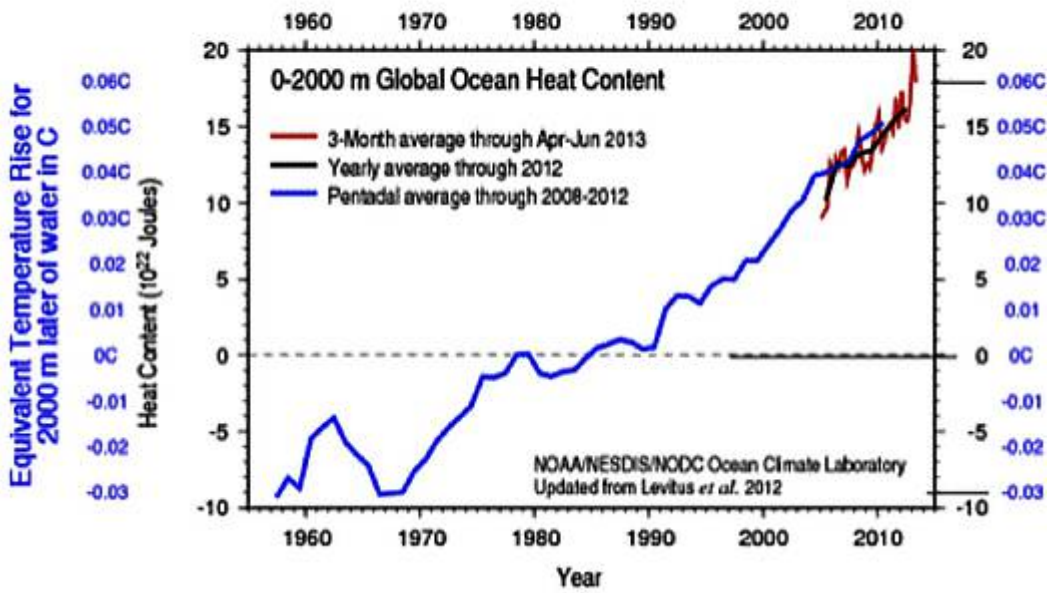
Abbildung 3: OHC-Veränderung der letzten 60 Jahre, ausgedrückt in Grad Celsius. Quelle: Lucia / The Blackboard .
