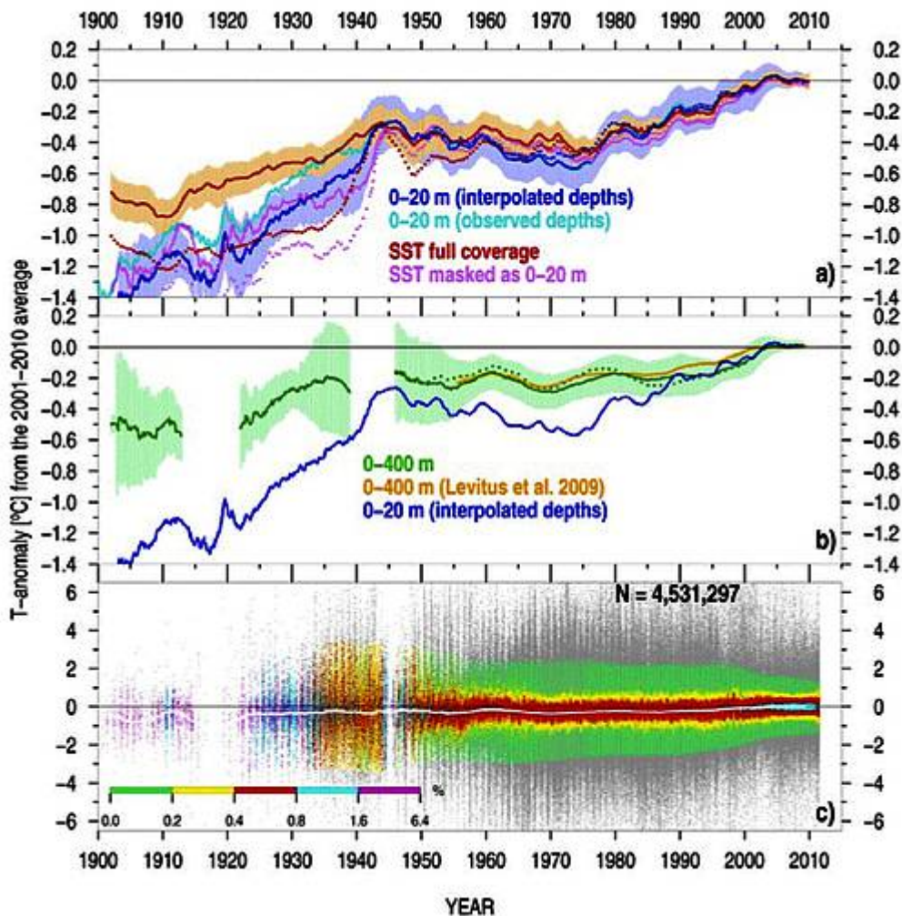
Abbildung 5: Entwicklung des globalen ozeanischen Wärmehalts für die letzten 110 Jahre nach Gouretski et al. 2012 . Grüne Kurve in Teilabbildung b zeigt OHC für das Tiefenintervall 0-400m.
