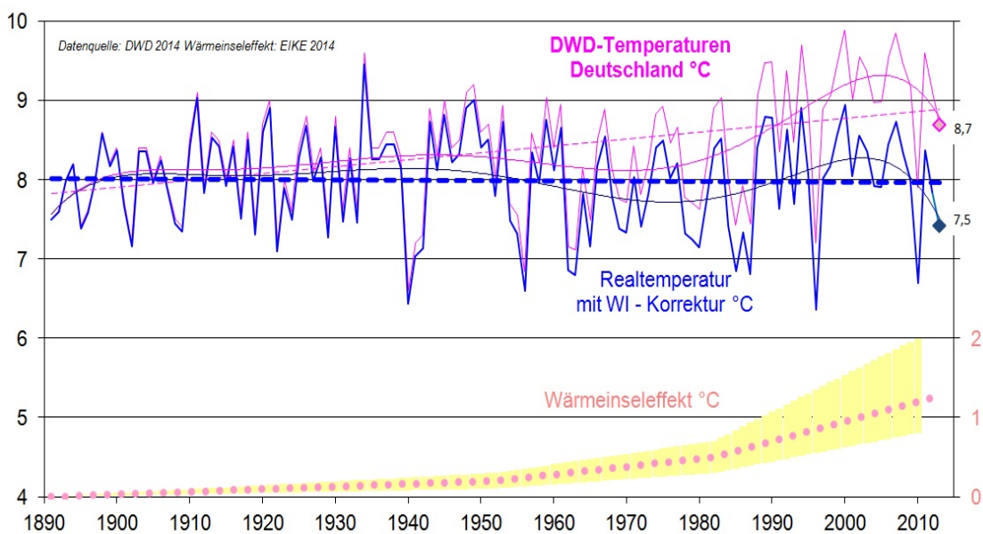
Die Deutschlandtemperaturen des DWD 1891 - 2013 - korrigiert um den Wärmeinsel-Effekt -
