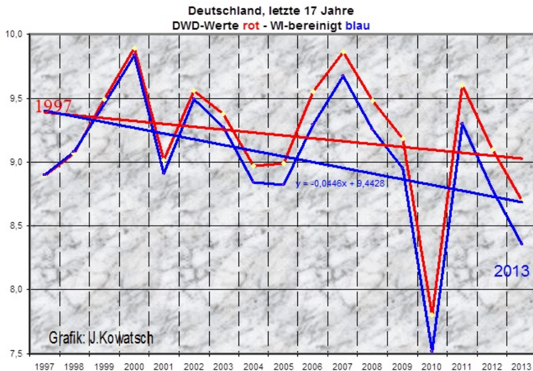
Abb 13: Die Deutschlandtemperaturen der letzten 17 Jahre. (Quelle: DWD-Werte Offenbach), mit und ohne WI-Betrachtung. Die von Excel errechnete Trendlinie sinkt um 0,7°C in den letzten 17 Jahren. Vorhergesagt war eine Erwärmung um +0,4°C.
