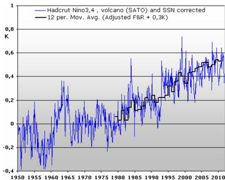
Abbildung 7: F&R beschreiben die Sonnenaktivität („TSI“, wie sie das nennen...) als von geringster Bedeutung in ihren Berechnungen. Jedoch ist es nur die Sonnenaktivität SSN, die dafür sorgt, dass Hadcrut selbst in den Jahren nach
