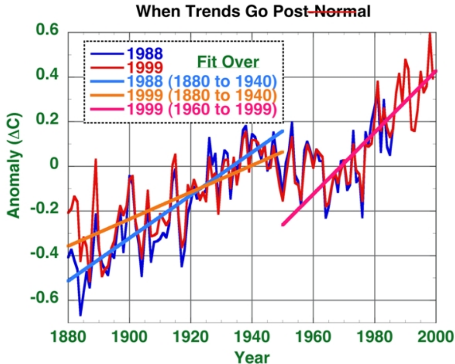
Abbildung 2: Die globalen jährlichen Temperaturtrends an der Erdoberfläche, wie sie 1988 und 1999 von GISS veröffentlicht worden waren. Blaue glatte Linie: Der Trend von 1880 bis 1940 aus dem Jahr 1988. Orange glatte Linie: Der Trend von 1880 bis 1940 nach den von GISS vorgenommenen Anpassungen der Daten. Rosa glatte Linie: die Rate von 1960 bis 1999. Dieser Trend verläuft auch eindeutig steiler als die Anomalien von 1988.
