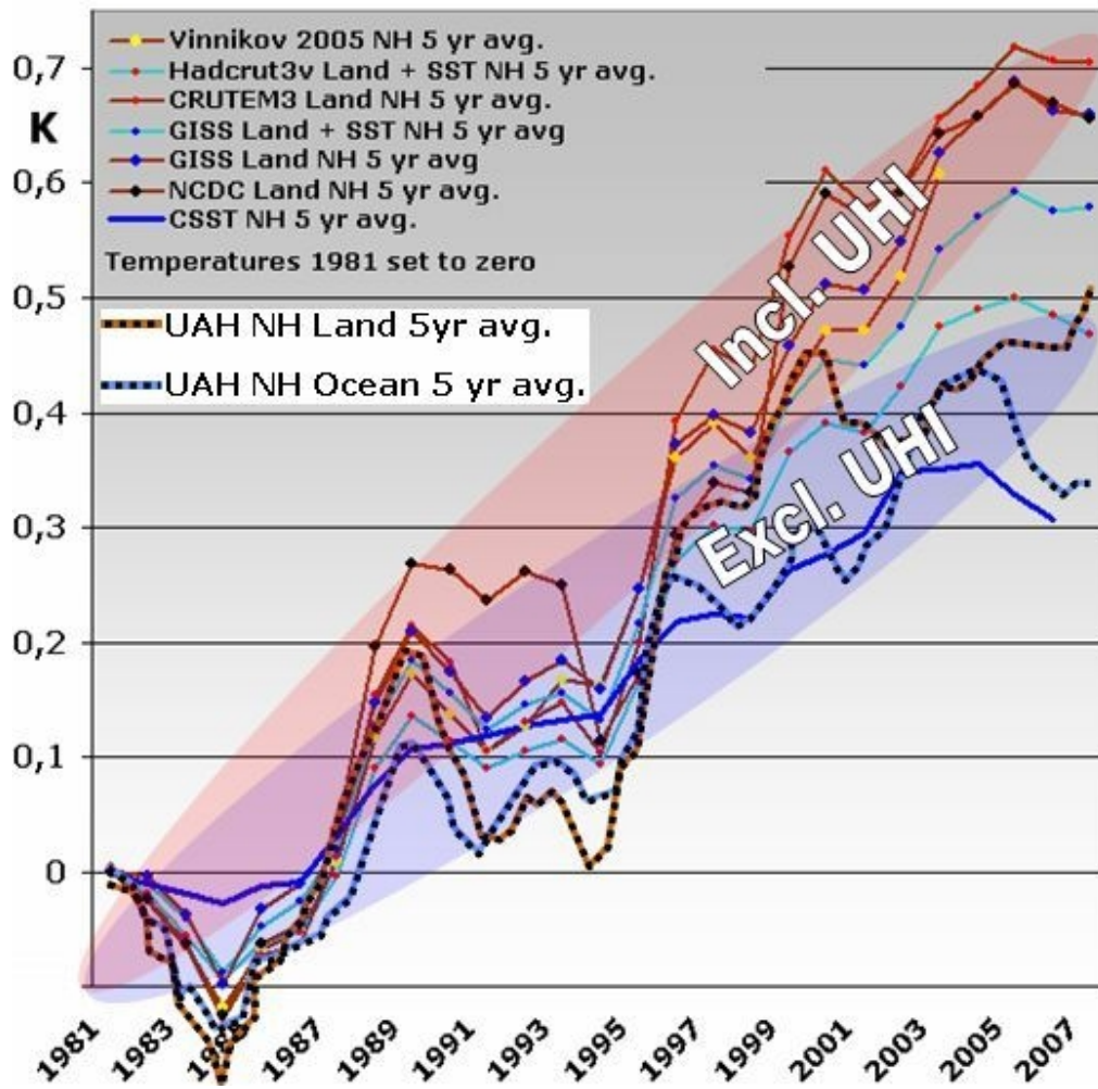
Abbildung 2: Hier spalten wir die Daten von der UAH nach Land und Wasser auf. Beide scheinen immer noch deutlich niedrigere Temperaturtrends zu zeigen als die Daten vom Land (braun), die zumeist in Städten und an Flughäfen am Boden gemessen werden.
