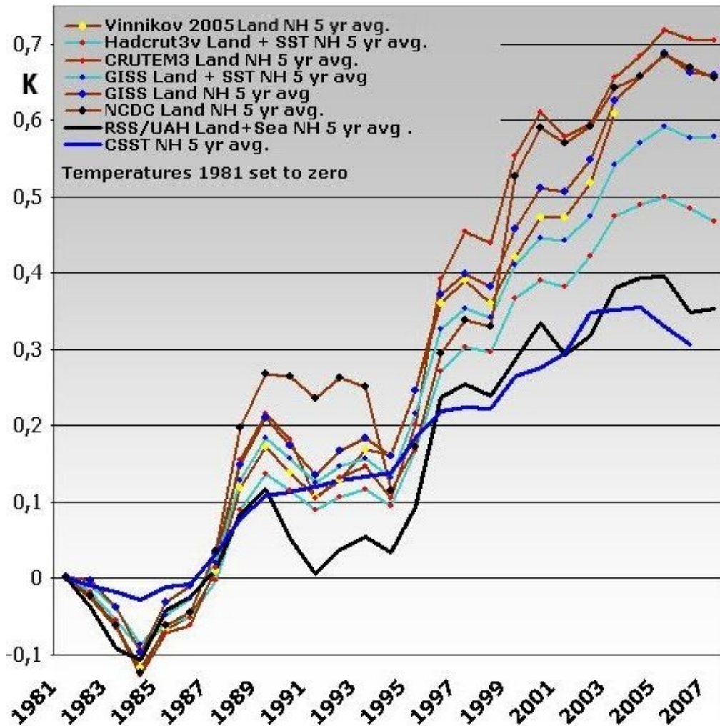
Abbildung 1: Der globale Temperaturtrend nach UAH gleicht den globalen Meerestemperaturen: Der schwarze Temperaturgraph – Mittel aus RSS + UAH-Satellitendaten der Nordhemisphäre (Land + Wasser) – zeigt einen geringeren Erwärmungstrend als der andere (braune) Graph, der nur die Entwicklung über Land zeigt – aber dem kühleren Verlauf der Wassertemperatur ähnelt. (Der blaue Graph ist ein Mittel ziemlich ähnlicher Aufzeichnungen der Wassertemperatur {SST}: MOHSST6, HADSST1, HASSST2, ERSST.v3b, HADISST1 und Kaplan SST 98.)
