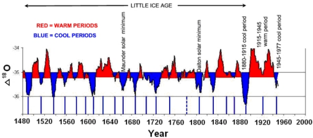
Abbildung 2. Erwärmung und Abkühlung von 1480 bis 1960.
