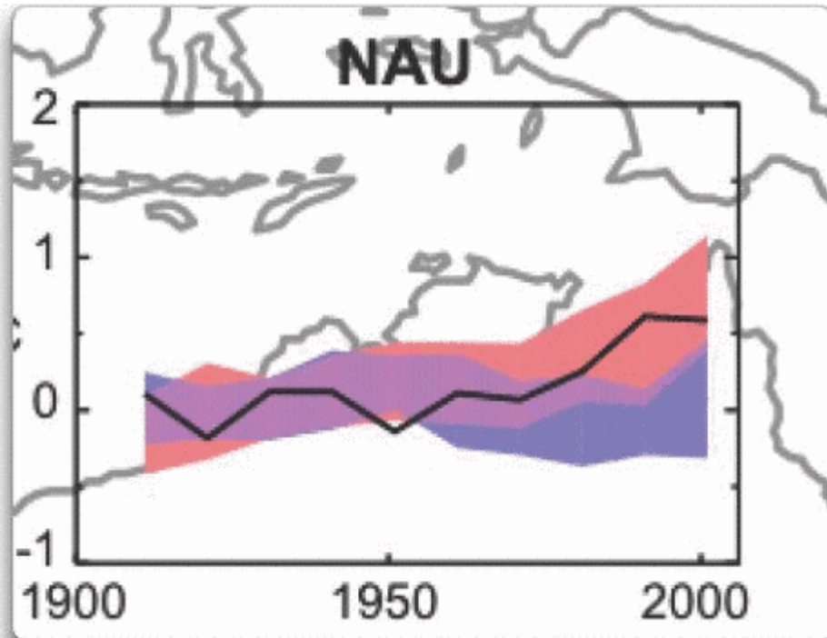
Abb. 1. Temperatur-Trends und Modellrechnungs-Ergebnisse für Nord-Australien. Die schwarze Linie sind die Messungen (Aus Fig. 9.12 des UN IPCC AR4). Betrifft das Gebiet von 110 Grad Ost bis 155 Grad Ost und von 30 Grad Süd bis 11 Grad Süd. Beruht auf den Landdaten von der CRU.
