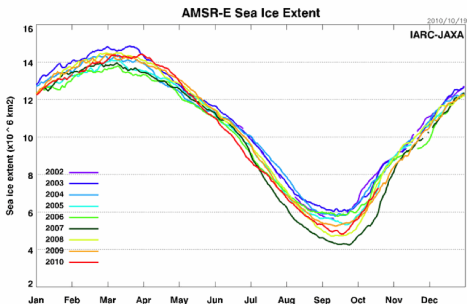
Abb. 1[1] : Arktische Eisbedeckung
