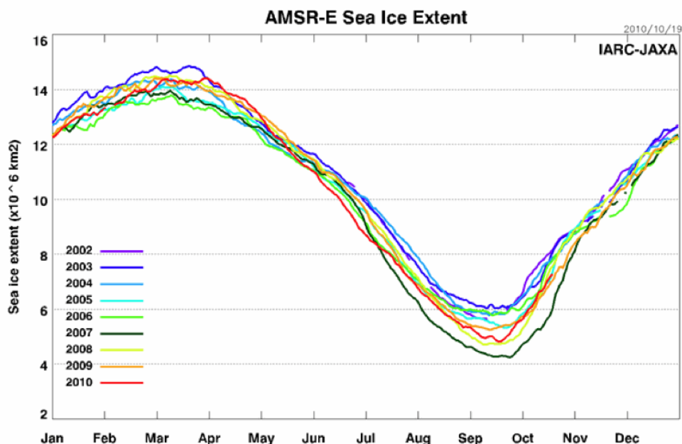
Abb. 1[1] : Arktische Eisbedeckung
