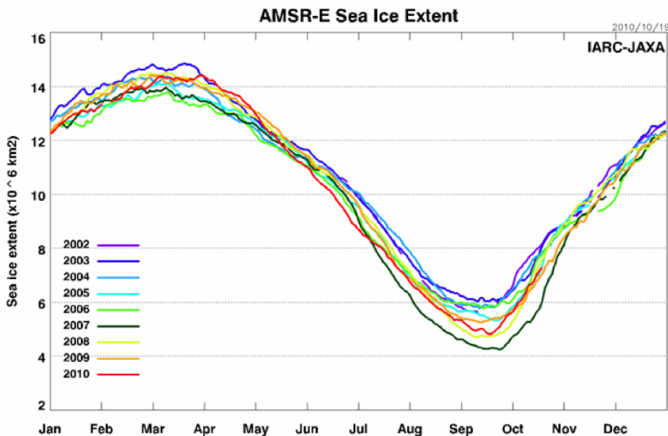
Abb. 1[1] : Arktische Eisbedeckung
