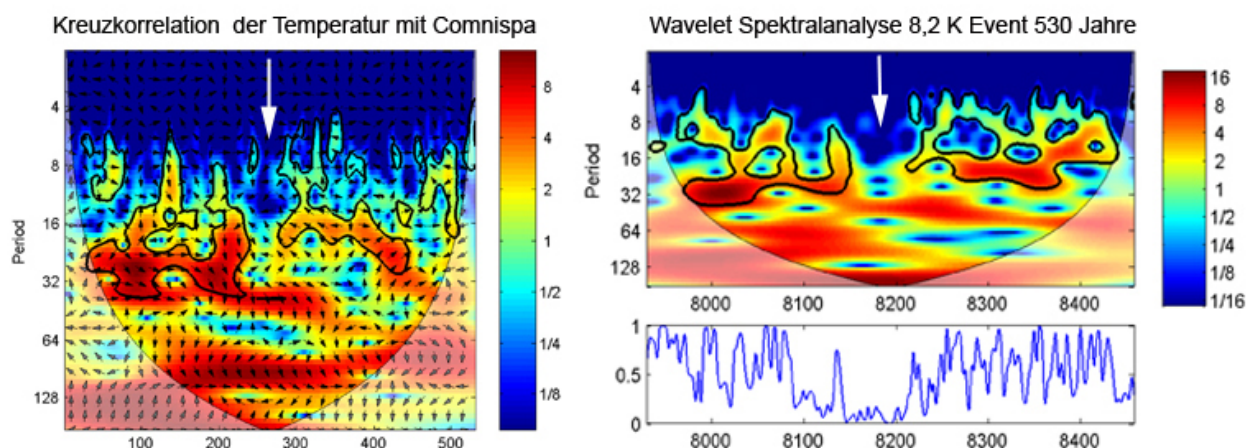
Abb. 10 Wavelet Spektralanalyse des 8,2 K Events. Links die spektrale Kreuzkorrelation eines 530 Jahre langen Temperaturverlaufs des 8,2 K Events mit der Comnispä-Zeitreihe. Rechts das CWT (continuous Wavelet Transform, Waveletspektrum) des 8,2 K Events. Die weißen Pfeile deuten den jeweiligen Temperatureinbruch an. Die Spektralfarben bedeuten die Spektralenergie in den Perioden. Dunkelblau: keine spektrale Energie, rot maximale Energie. Die fett umrandeten Bereiche sind 95 %
