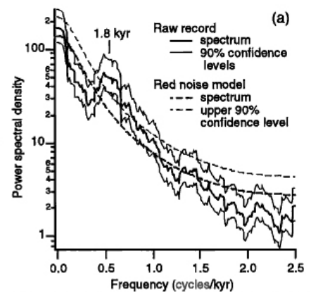
Abb. 6 a) Dansgaard-Öeschger-Schwankungen in den letzten 100 000 Jahren, MTM-Spektralanalyse der D/O-Zyklen mit signifikantem 1800 Jahre-Zyklus im Mittel. [3]
