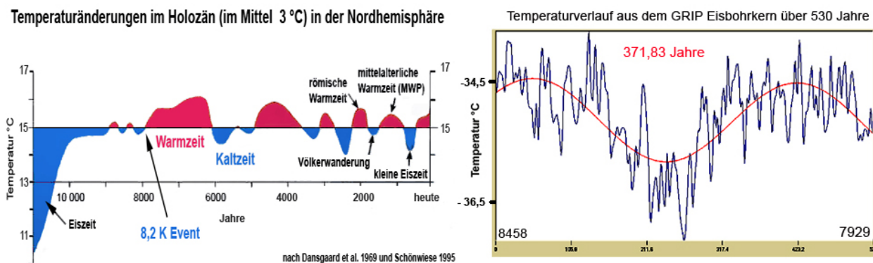
Abb. 9 Temperaturverlauf im Holozän auf der Nordhemisphäre (links) und rechts die aus dem GRIP Eisbohrkern rekonstruierte Temperatur seit 8458 Jahren bis vor 7929 Jahren (530 Jahre) [10, Beck 2010].
