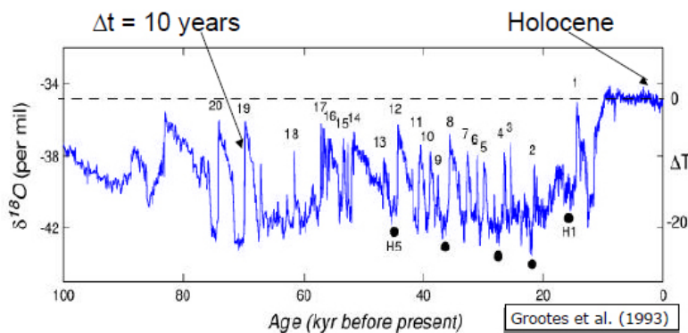
Abb. 6 a) Dansgaard-Öeschger-Schwankungen in den letzten 100 000 Jahren, MTM-Spektralanalyse der D/O-Zyklen mit signifikantem 1800 Jahre-Zyklus im Mittel. [3]
