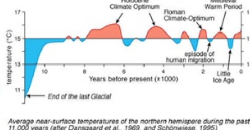
Temperaturschwankungen im Holozän (im Mittel 3 °C)
