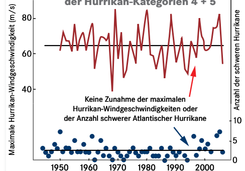
Abb. 7) Anzahl und maximale Windstärke der Hurrikan-Kategorien 4 + 5
