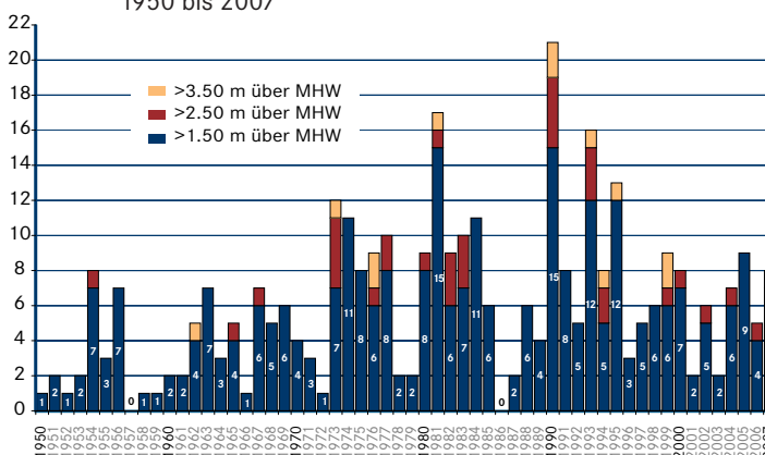
Abb. 3) Häufigkeit der Sturmfluten in Hamburg 1950 bis 2007
