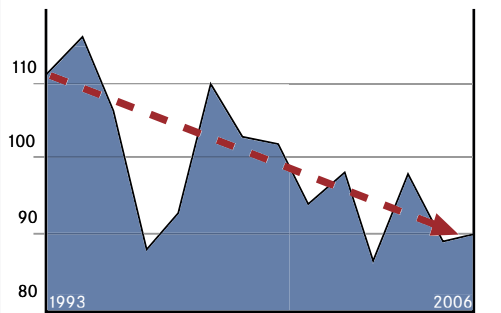
Abb. 5) Winderträge zum langjährigen Mittel in %
