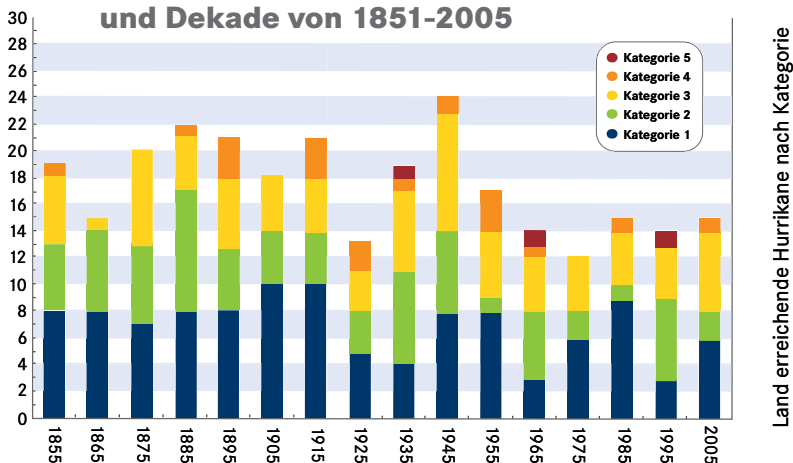
Abb. 6) USA Land erreichende Hurrikane nach Kategorie und Dekade von 1851-2005
