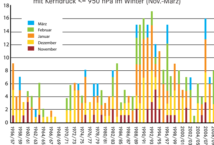
Abb. 2) Anzahl nordatlantischer Orkantiefs mit Kerndruck <= 950 hPa im Winter (Nov.-März)
