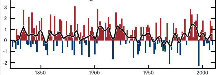
Abb. 1) NAO Index Winter 1820-2009:
