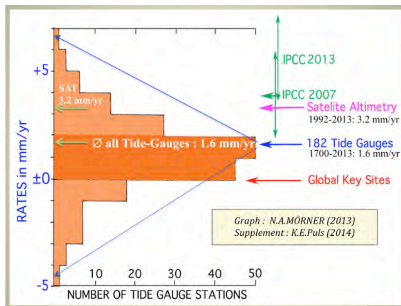
Abbildung 8: GAUSS-Verteilung 182 Pegel [10]
